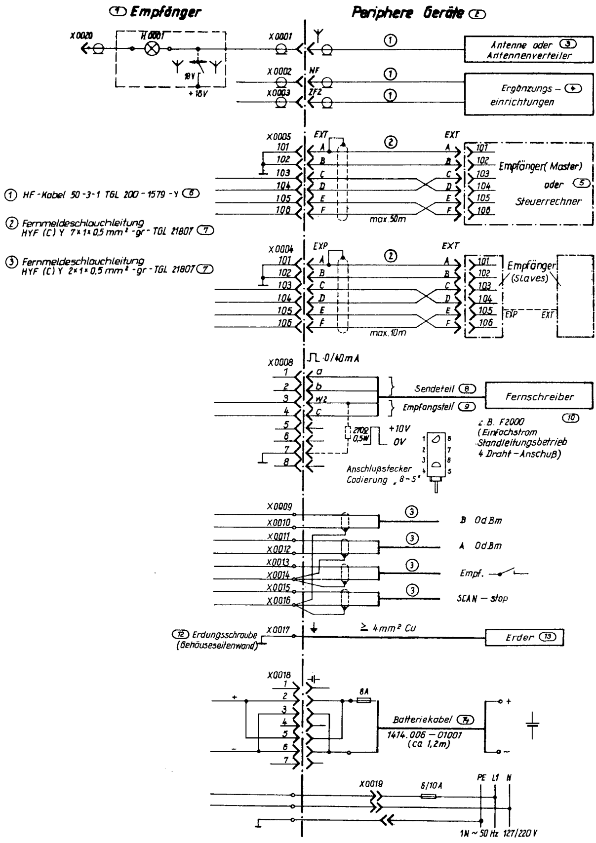
Anschlußplan 1340.042-00001 Ap
